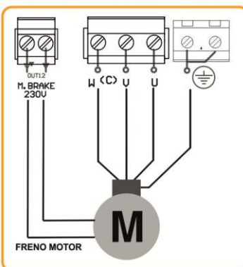
MOTOR TRIFÁSICO 400V
