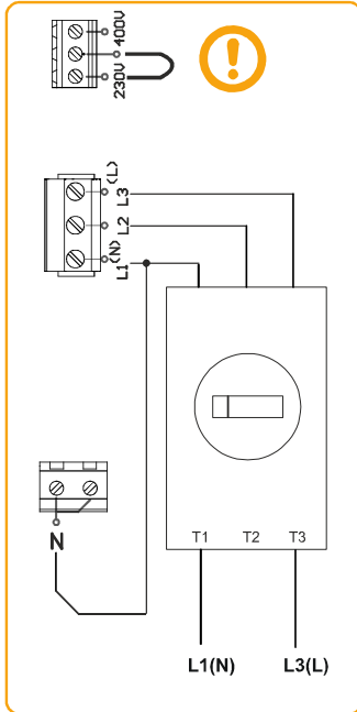
ALIMENTACIÓN 230V
