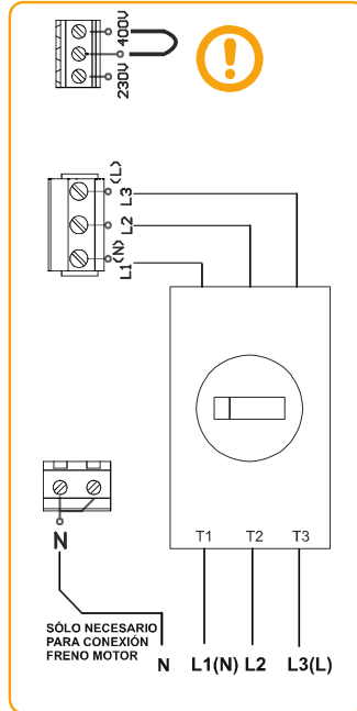
ALIMENTACIÓN 400V
