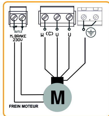
MOTEUR MONOPHASE 230V MOTEUR TRIPHASE 400V
