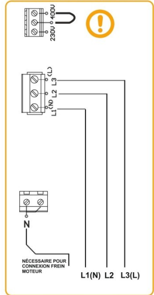
ALIMENTATION 400V TRIPHASE
