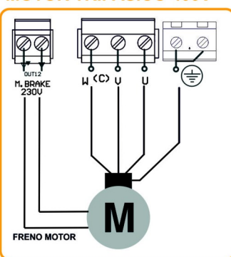
MOTOR TRIFÁSICO 400V
